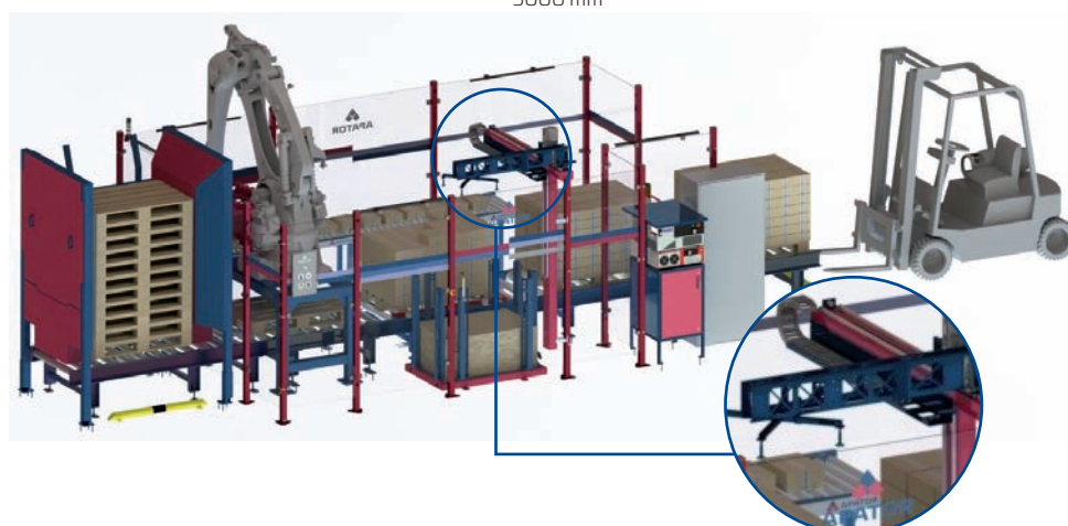
Manipulator przekładek
